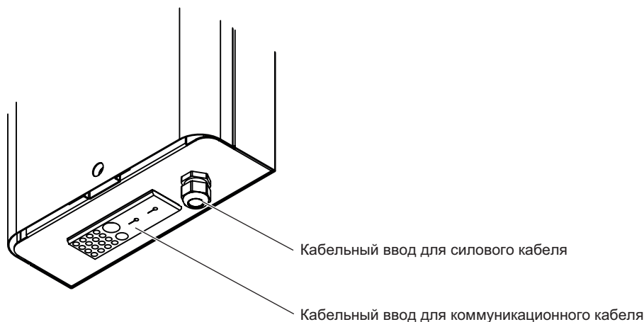
Рис. 20. Ввод кабелей
