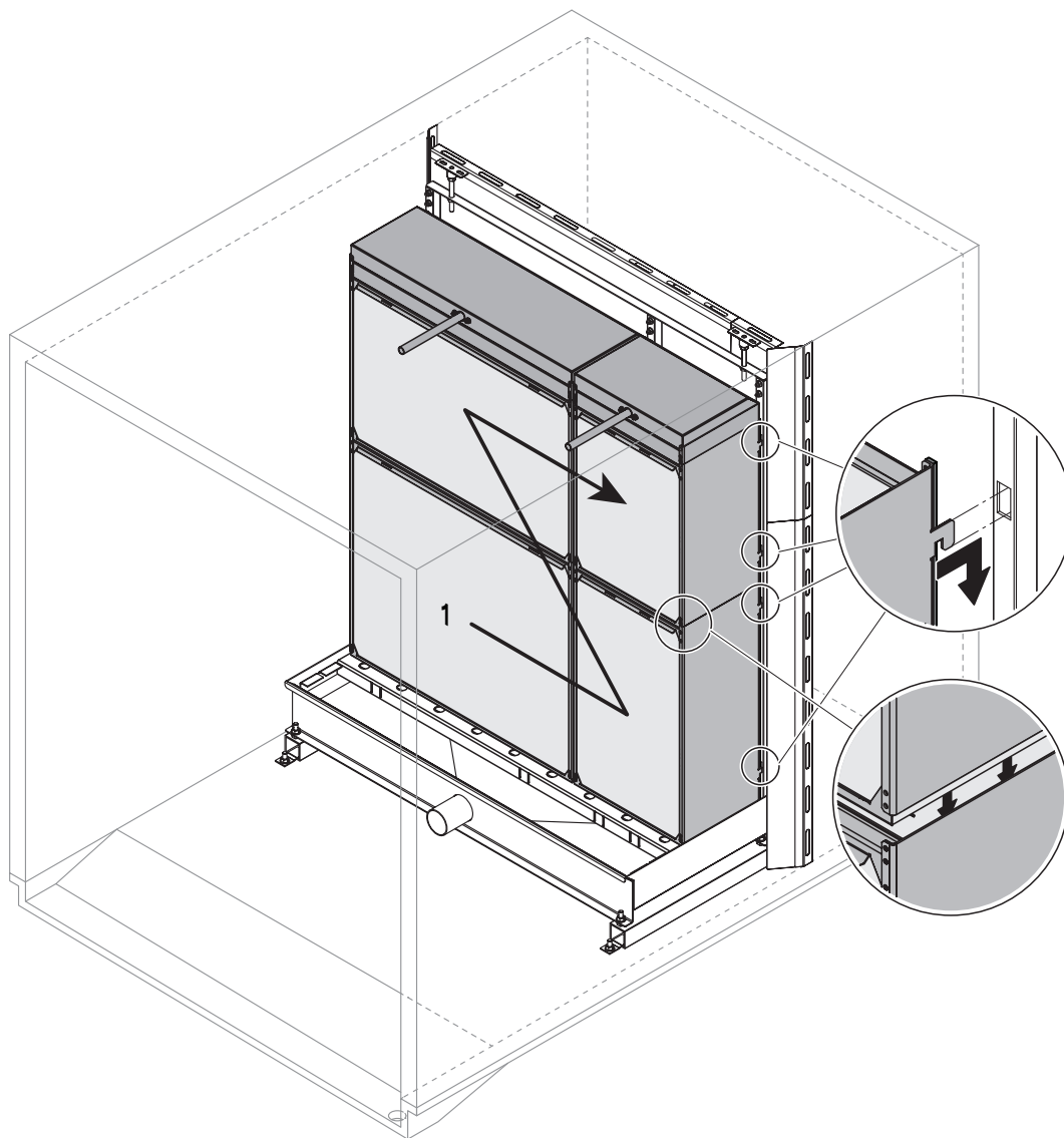
Рис. 11. Монтаж насадок
