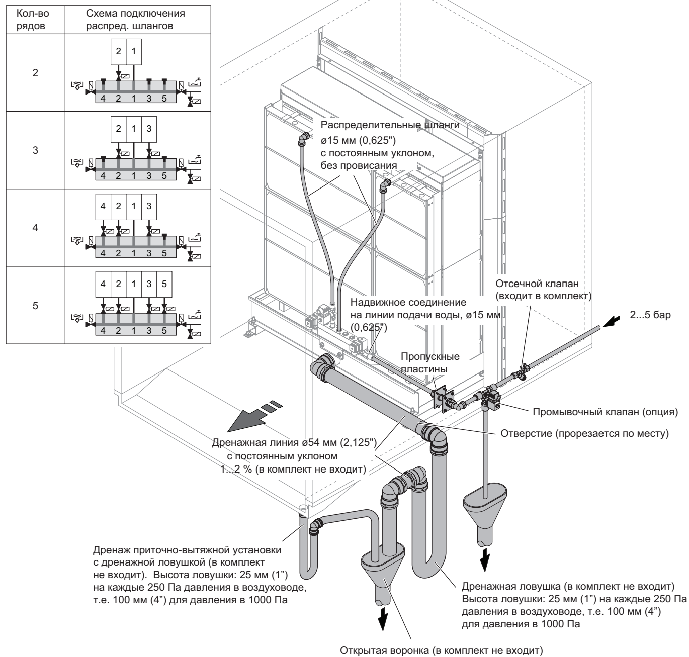
Рис. 17. Подключение линий воды ME Direct Feed (внутренний монтаж)
